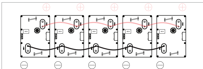
Figure 7. Branchements négatifs en parallèle
