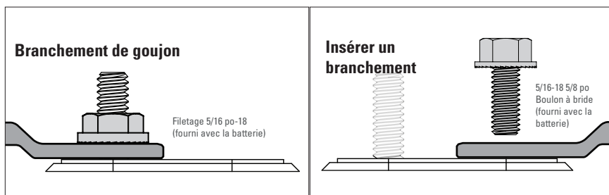
Figure 5. Bonne installation de la borne.
