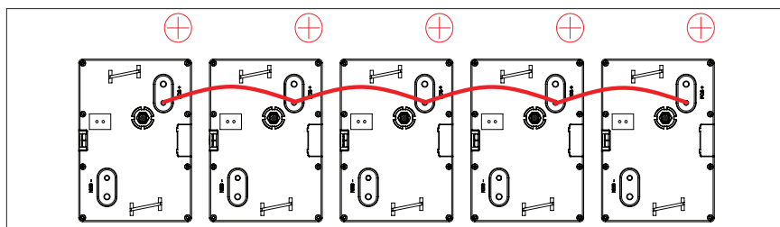
Figure 6. Branchements positifs en parallèle
