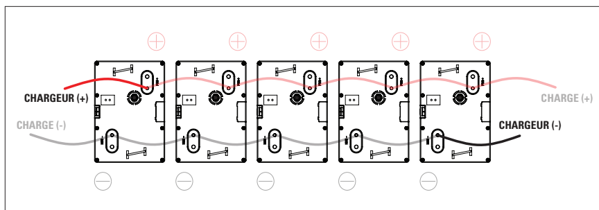
Figure 9. Branchements de chargeur
